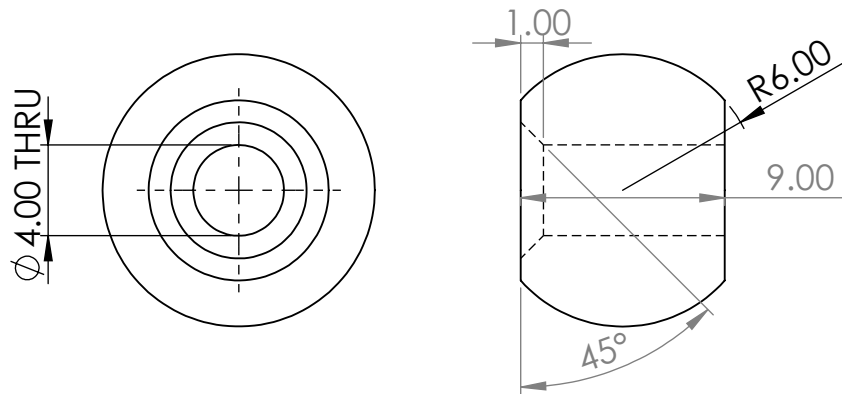
Bar Globe
